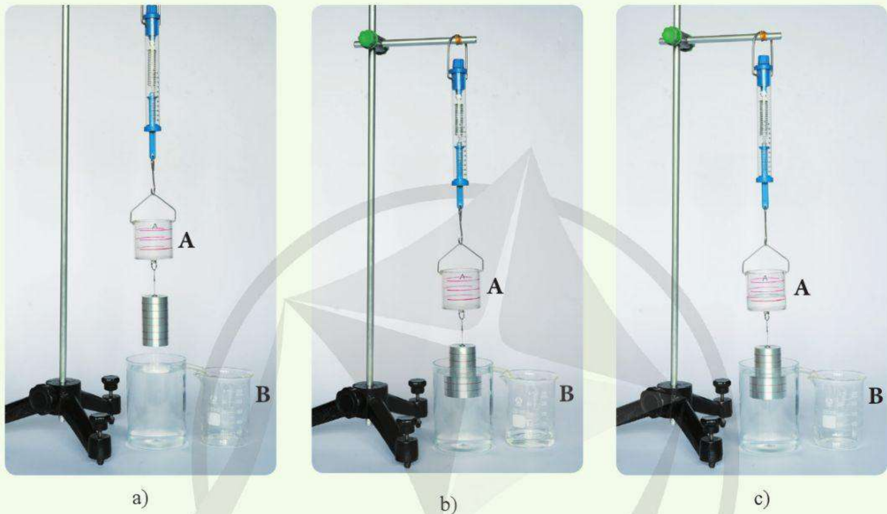
Hình 15.5. Thí nghiệm xác định độ lớn của lực đẩy Acsimet
