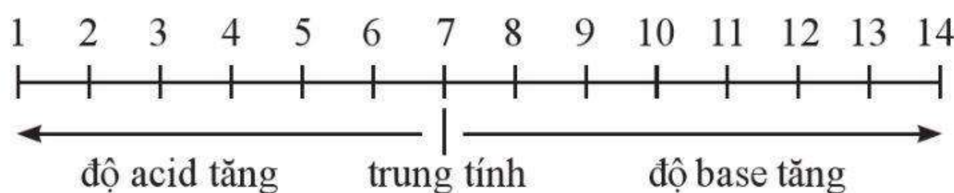
Hình 10.3. Thang pH
