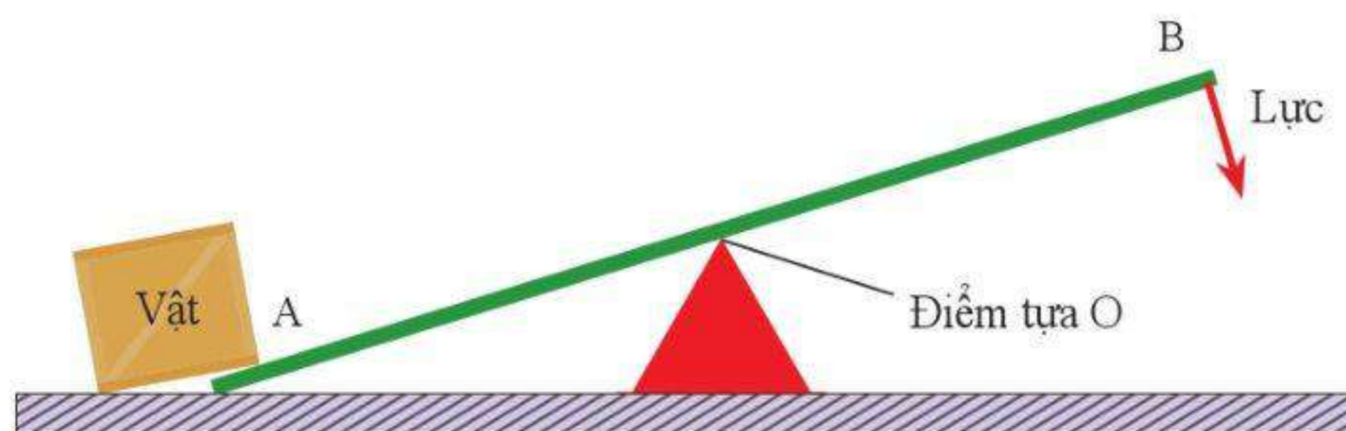
Hình 19.3. Mô hình đòn bẩy đơn giản
