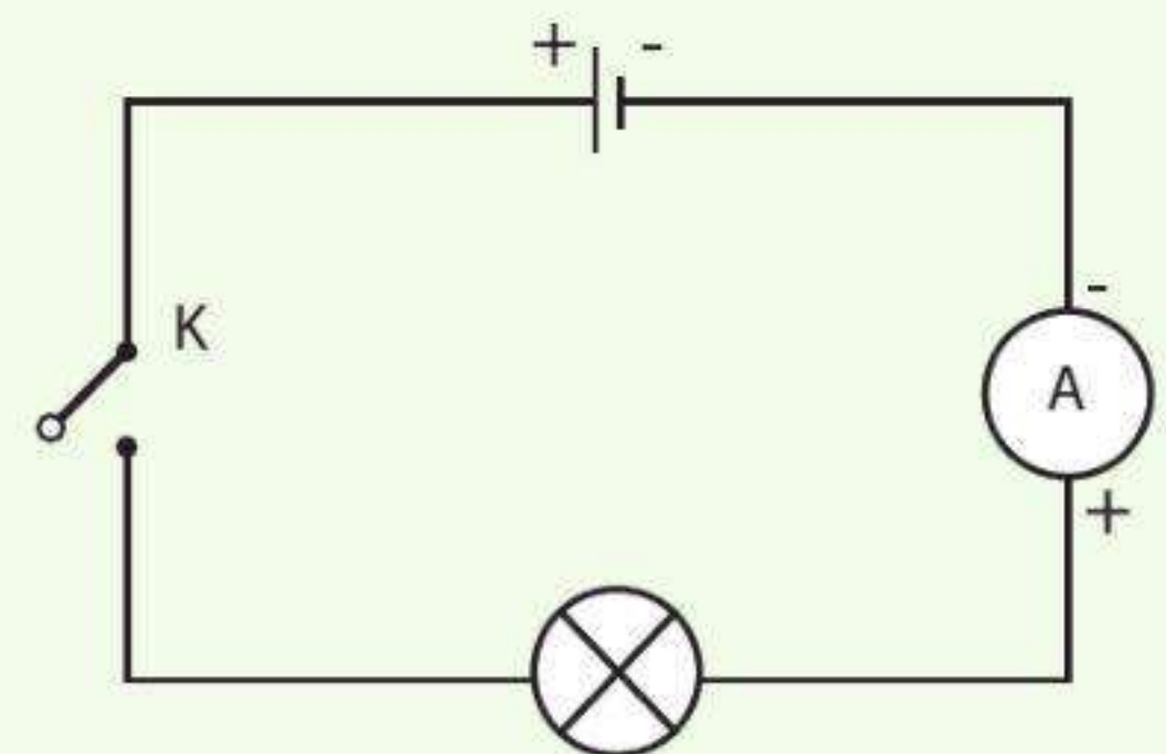
Hình 23.2. Sơ đồ mạch điện đo cường độ dòng điện
