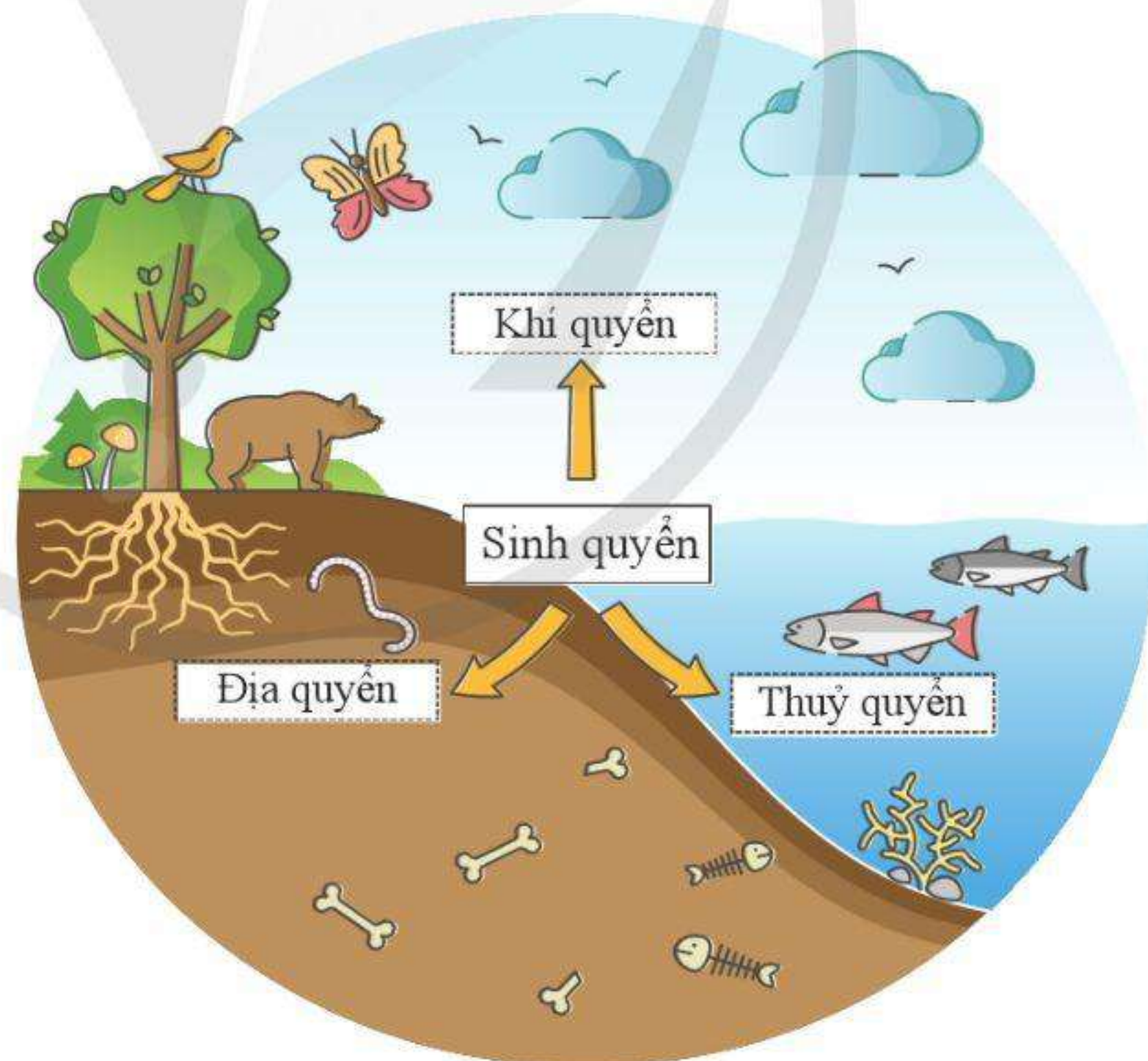
Hình 43.1. Sinh quyển
